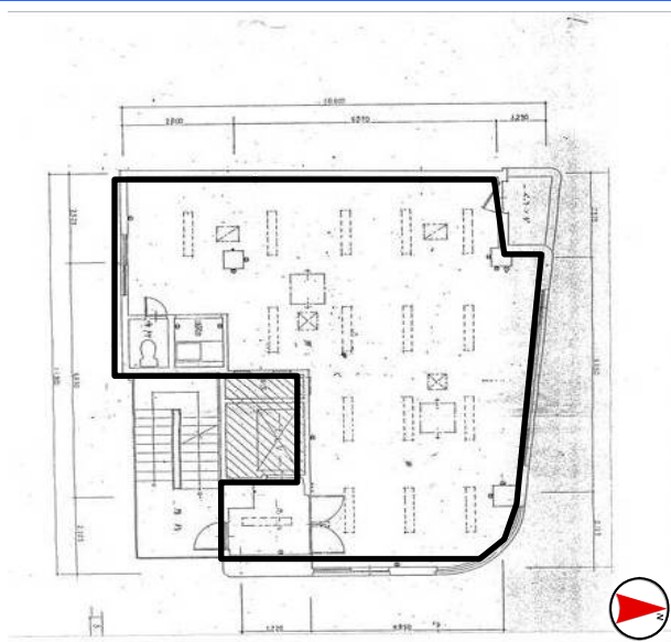
6階 平面図
